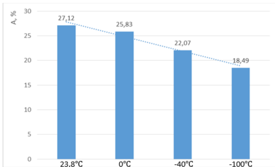
Slika 5.4. Histogram istezljivosti mekog čelika
