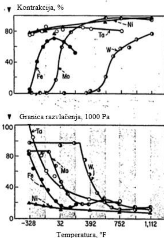
Slika 3.8. Promjena istežljivosti (gornja slika) i granice razvlačenja (donja slika) u odnosu na snižavanje temperature za tehnički čiste materijale sa BCC rešetkom i Ni sa FCC rešetkom [7]
