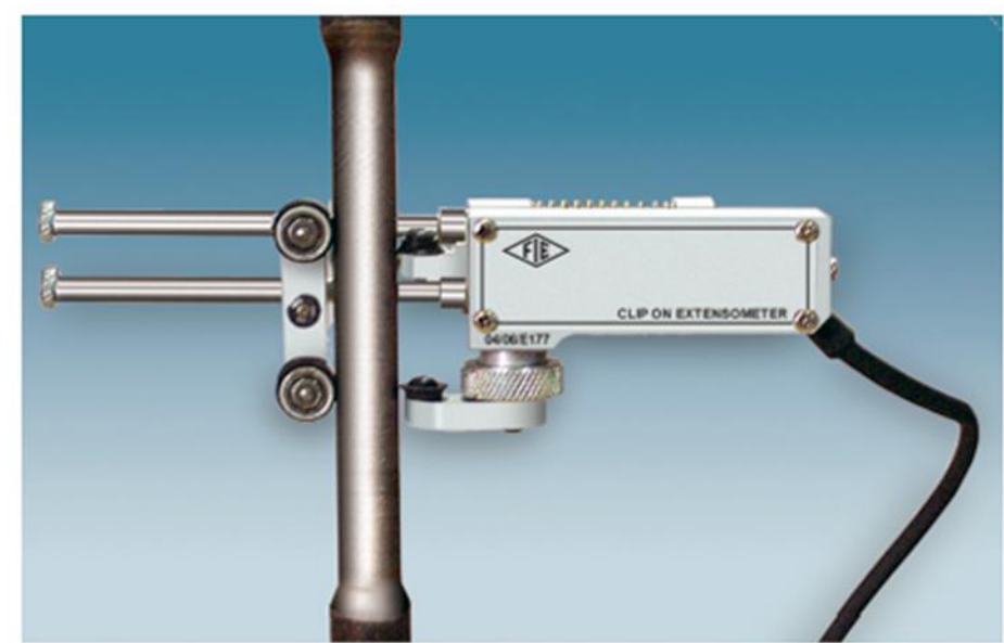
Slika 2.5. Nasadni ekstenzometar
