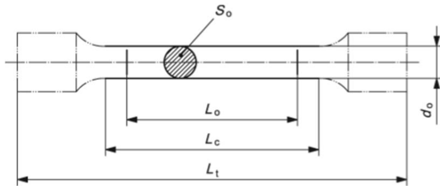
Slika 2.9. Skica okrugle epruvete
