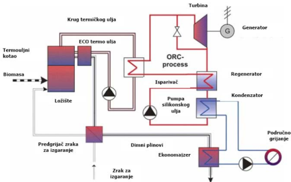
Slika 19. Shema ORC kogeneracijskog postrojenja na biomasi [12]
