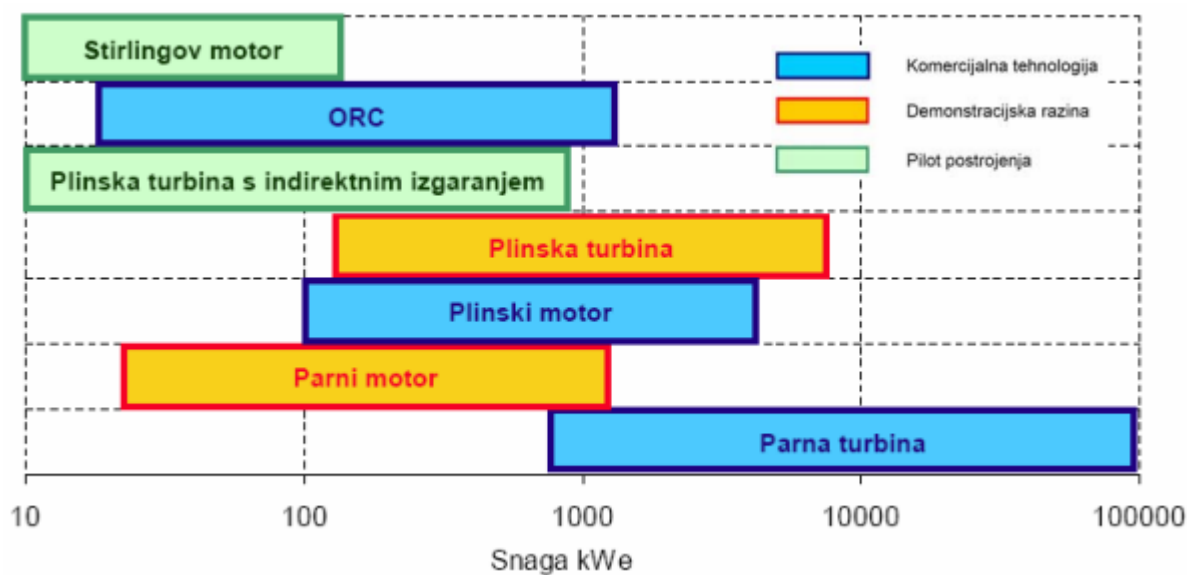
Slika 18. Tržišni status različitih tehnologija kao i raspon primjena s obzirom na veličinu kogeneracijskog postrojenja [12]
