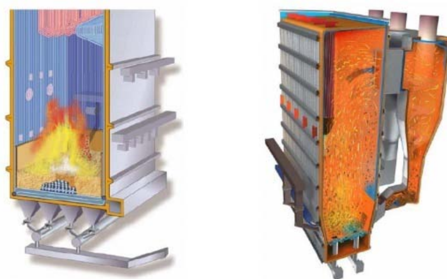
Slika 16. Presjek ložišta s izgaranjem u fluidiziranom sloju: mjehurićasti (lijevo) i cirkulirajući (desno) [21]
