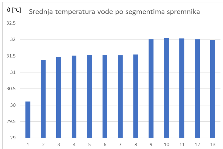
Slika 22. Dijagram uprosječene inicijalne temperature po segmentima spremnika u zimskom režimu rada koje su dobivene računalnom simulacijom
