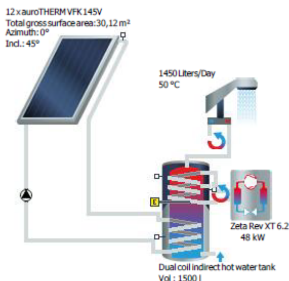
Slika 36. Prikaz komponenta i način spajanja na spremnik PTV-a
