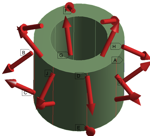
Slika 6.9. Rezultantne sile na vanjskoj stijenci namota
