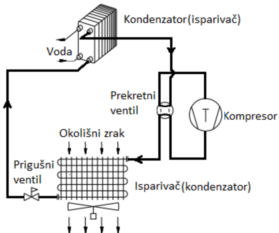
Slika 8. Rad uređaju u procesu odleđivanja isparivača [5]
