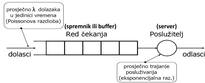
Slika 23. Struktura modela čekanja [31]
