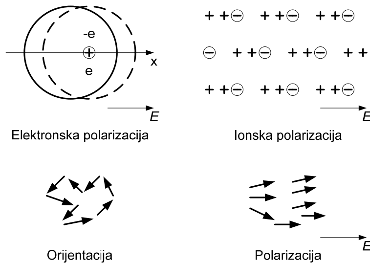
Slika 2.8. Proces polarizacije [2]
