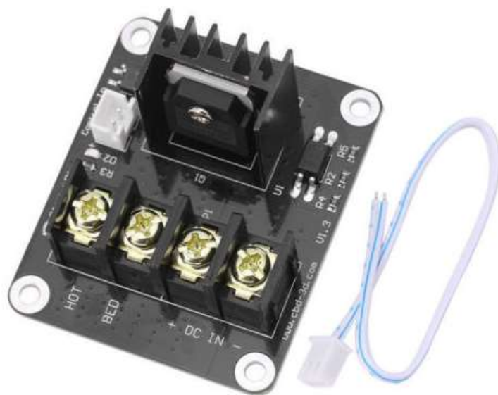
Slika 10. MKS MOSFET
