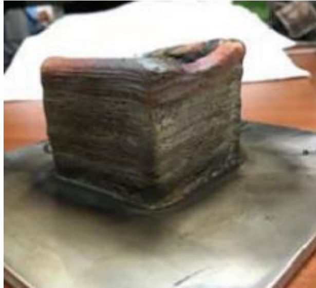
Slika 6. Komponenta od austenitnog nehrđajućeg čelika izrađena WAAM postupkom [15]
