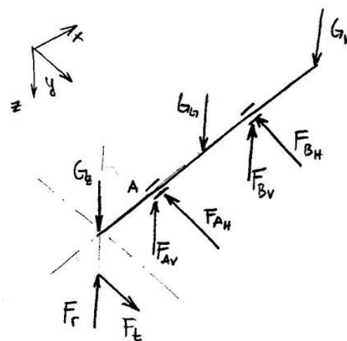
Slika 12. Vratilo sa silama opterećenja u izometriji
