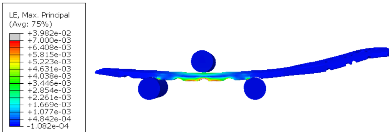
Slika 26. Deformacije pločice
