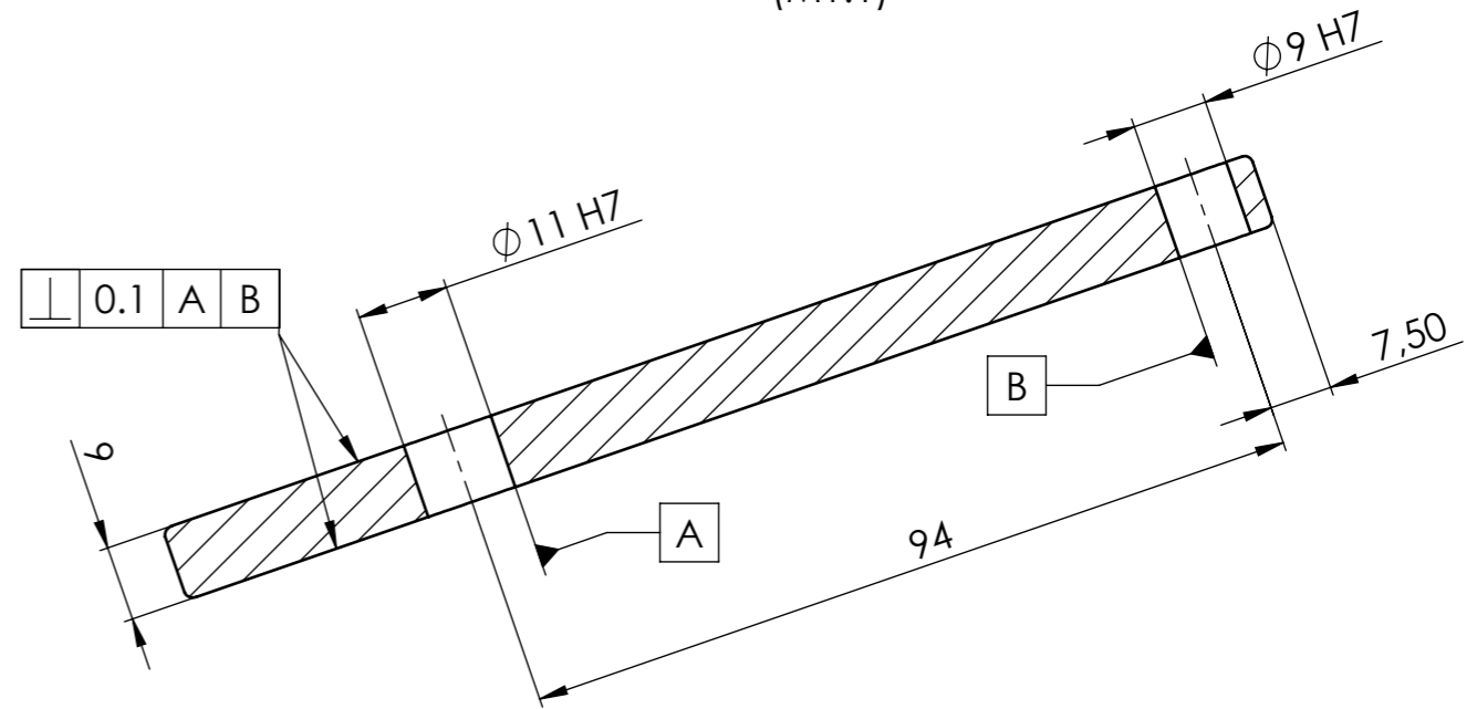
A-A (M1:1)
