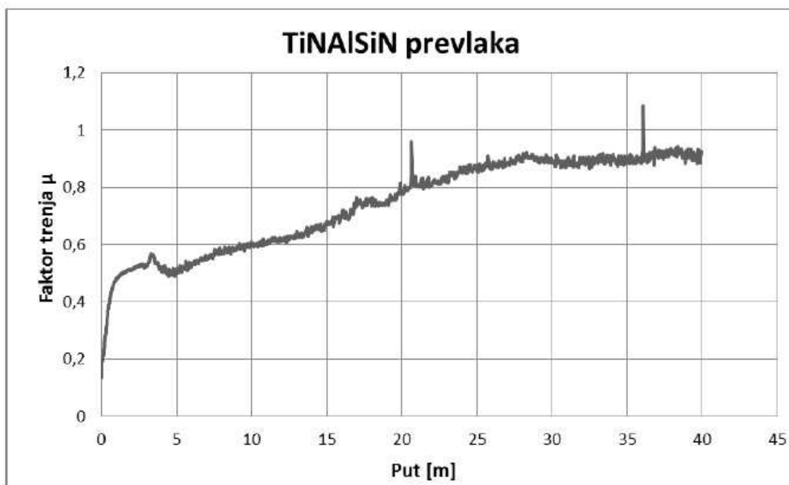
Slika 37. Ovisnost koeficijenta faktora trenja o prijedenom putu za TiNAlSiN prevlaku [9]
