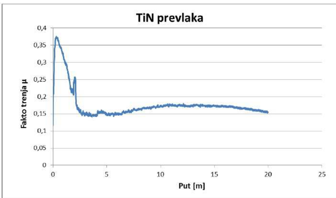
Slika 38. Ovisnost koeficijenta faktora trenja o prijedenom putu za TiN prevlaku [9]
