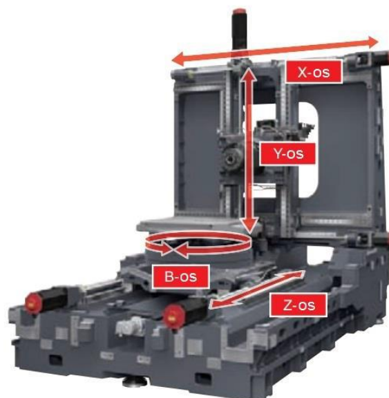
Slika 10. Horizontalni glodači obradni centar [12]
