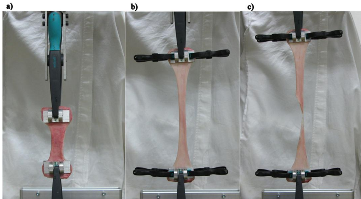
Slika 34 Vlačno ispitivanje uzoraka do pucanja: a) uzorak pozicioniran u prihvatima, b) uzorak tijekom opterećivanja i c) uzorak neposredno prije pucanja
