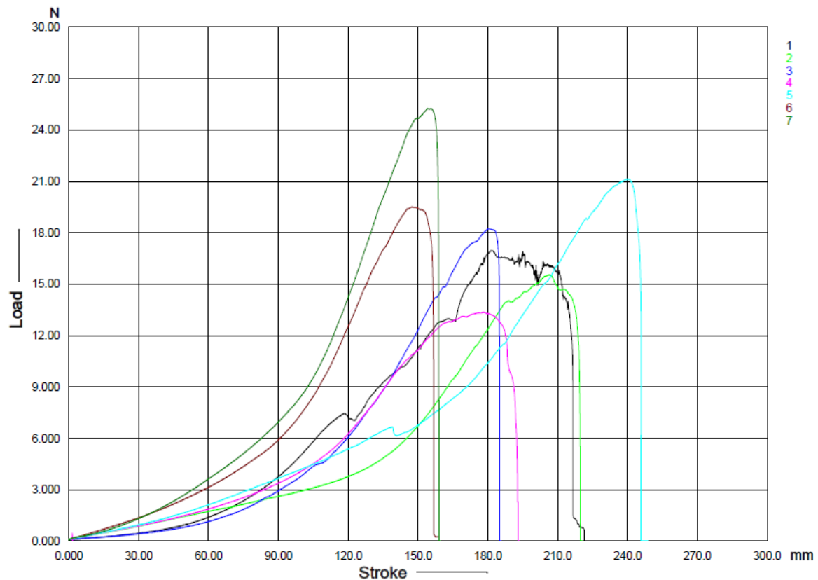
Slika 39 Dijagram sila-pomak za uzdužne uzorke
