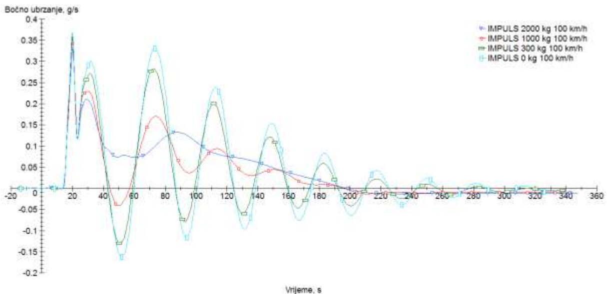
Slika 80. Bočno ubrzanje za različite iznose mase tereta, CarSim
