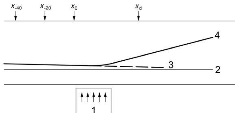
Slika 30. Ispitna staza [15]
