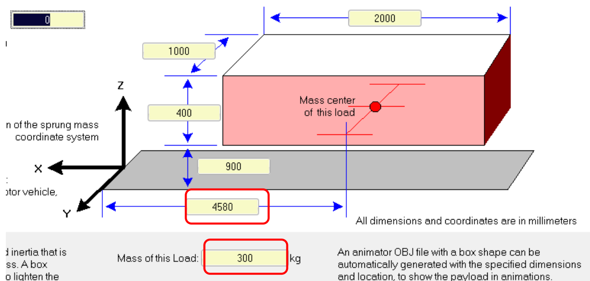
Slika 43. Masa tereta, CarSim
