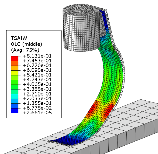
Slika 35. Raspodjela iznosa za Tsai-Wu kriterij u zadnjem sloju treće varijante u trenutku t = 0.112 s
