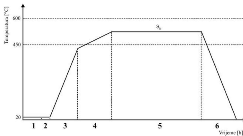
Slika 9 Shema postupka plazmatskog nitriranja [10]
