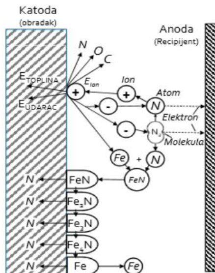
Slika 6 Koebel-ov model nitiranja u plazmi [10]
