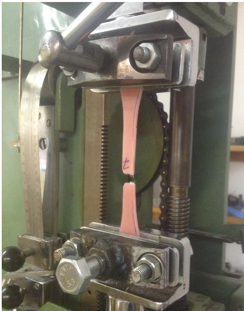
Slika 29. Lom epruvete u prvom ciklusu ispitivanja statičkog vlačnog pokusa
