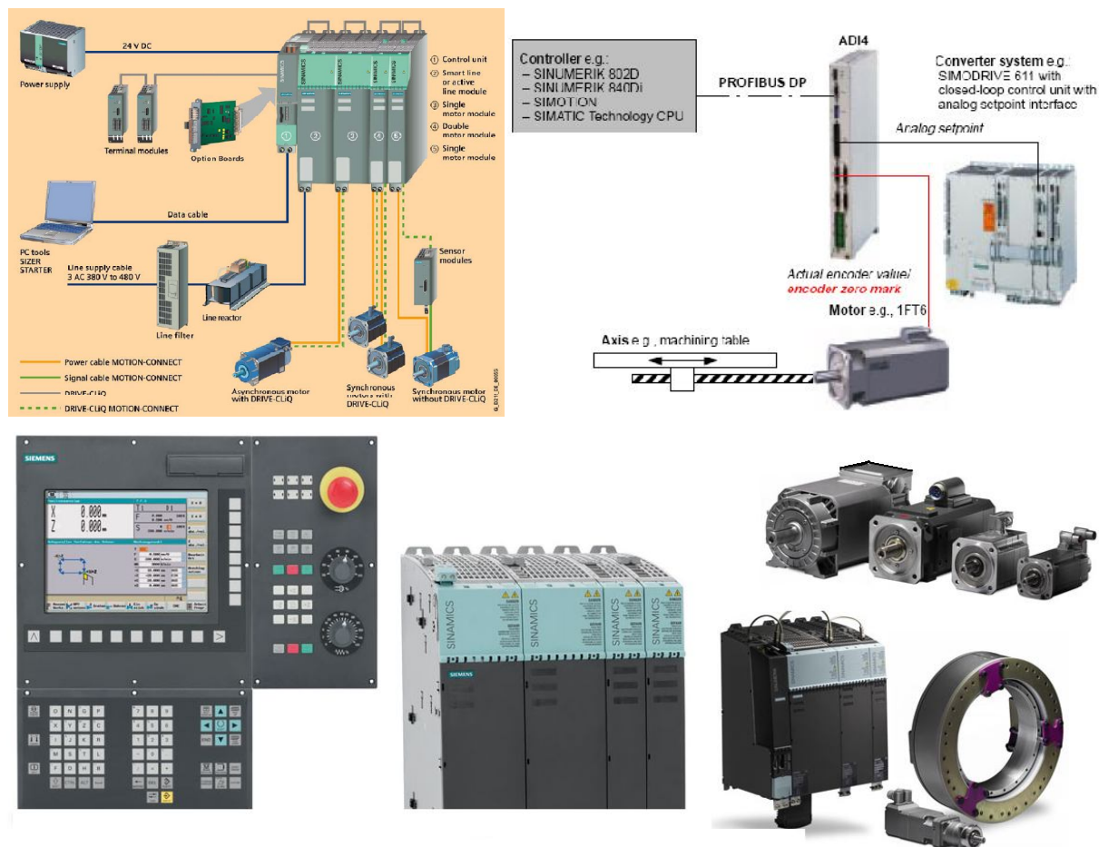
Slika 21. Siemensov upravljački sustav [24]
