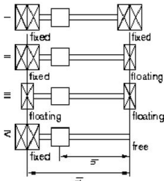
Slika 32. Načini uležištenja kugličnog navojnog vretena
