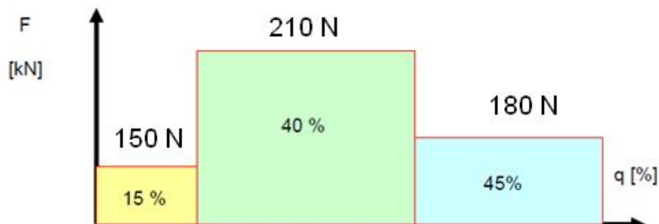
Slika 49. Dinamička opterećenja na KNV, Z –os, F - q
