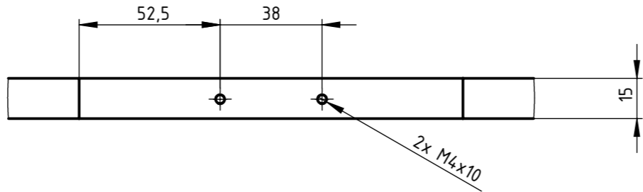
A mjerilo 1:2
