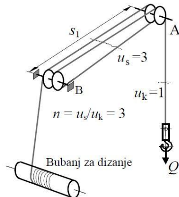
Slika 9. Koncept 1 - prikaz koloturnika za kompenzaciju užeta [8]
