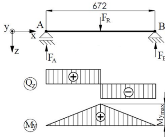
Slika 47. Dijagrami opterećenja osovine skretnih užnica na dohvatniku
