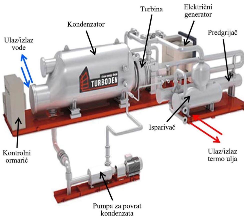
Slika 6. Turboden 10 CHP-Split [8]
