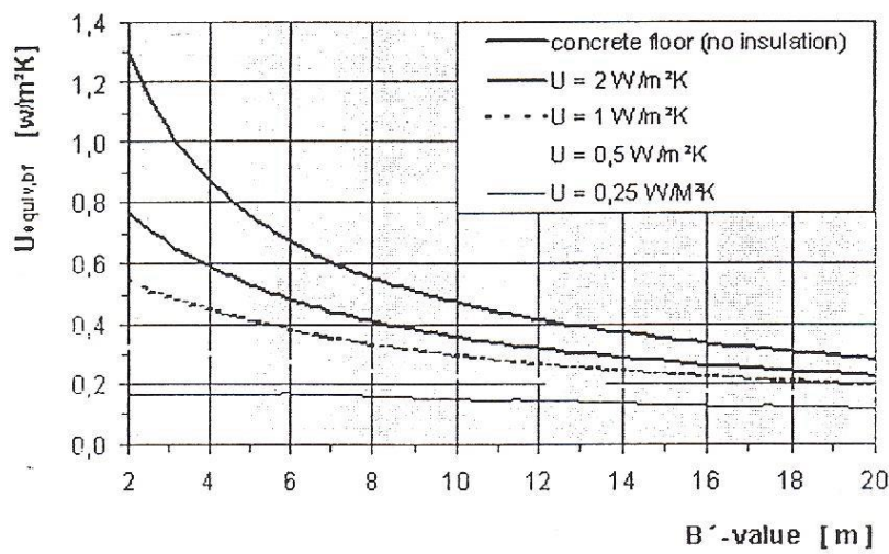
Slika 4. Ekvivalentni koeficijent prolaza topline kao funkcija koeficijenta prolaza topline poda i vrijednosti B'
