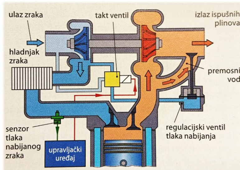
Slika 31. Elektonička regulacija obilaznog ventila [27]
