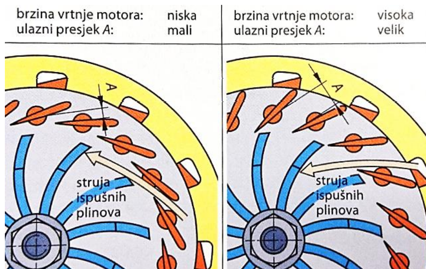
Slika 33. Namještanje statorskih lopatica [27]
