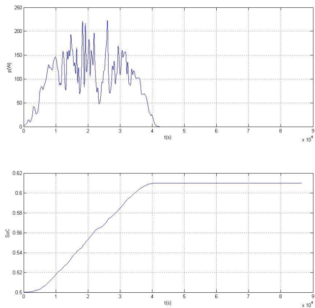
Slika 43 Stanje napunjenosti baterije u slučaju ispada trošila
