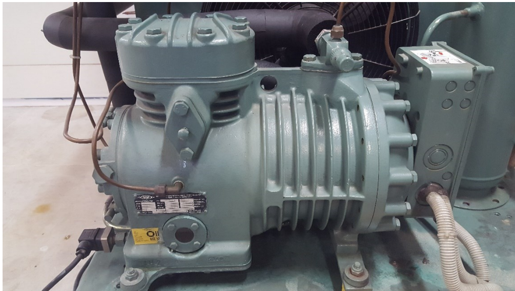
Slika 14. Kompresor
