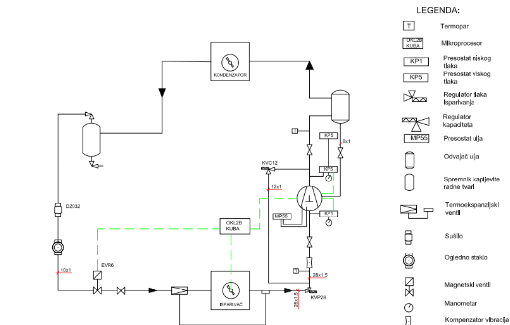
Slika 15. Shema mjerne linije
