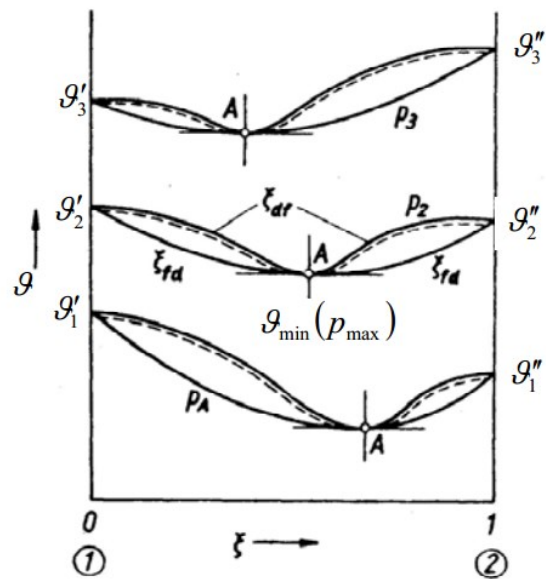
Slika 6. Azeotropska smjesa s temperaturnim minimumom vrenja [4]
