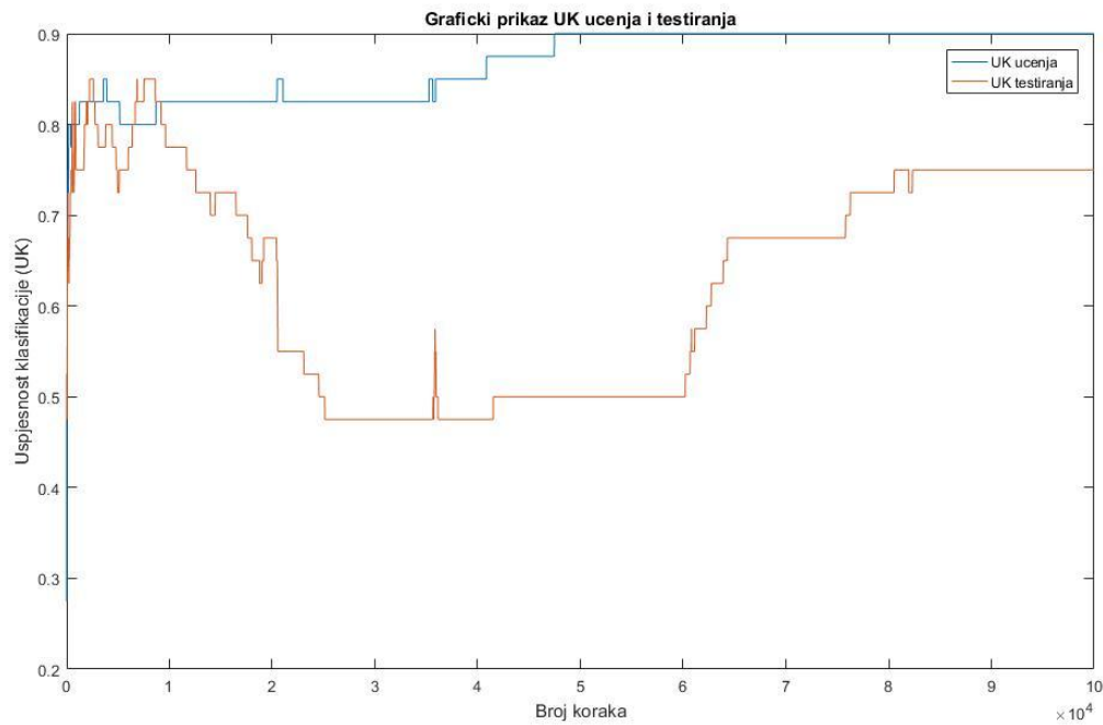
Slika 5.12. Grafički prikaz UK kod svih značajki pri \eta = 0.025 , \alpha = 0.05 n_{skriivenih} = 3
