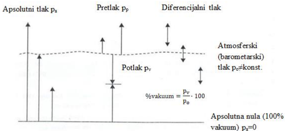
Slika 1. Odnos tlakova [3]
