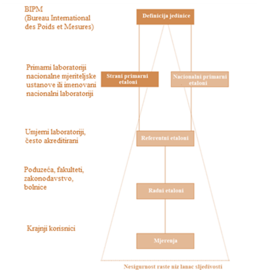
Slika 8. Lanac sljedivosti
