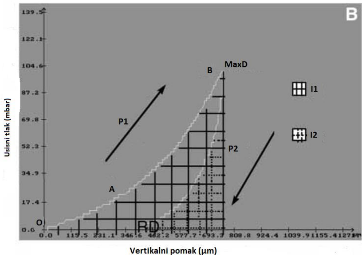
Slika 4.4. Dijagram ovisnosti vertikalnog pomaka i usisnog tlaka [19]
