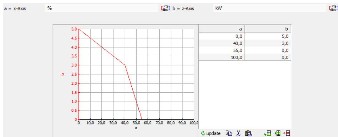
Slika 3.6. Mapa snage alternatora
