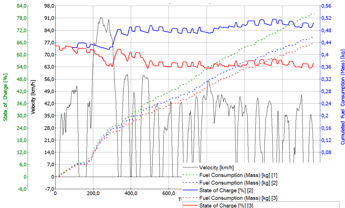
Slika 5.14. Usporedba trajektorija SoC-a i potrošnje goriva na UDSS voznom ciklusu za tri konfiguracije: [1] Konvencionalna, [2] Hibridna bez SA, [3] Hibridna sa SA
