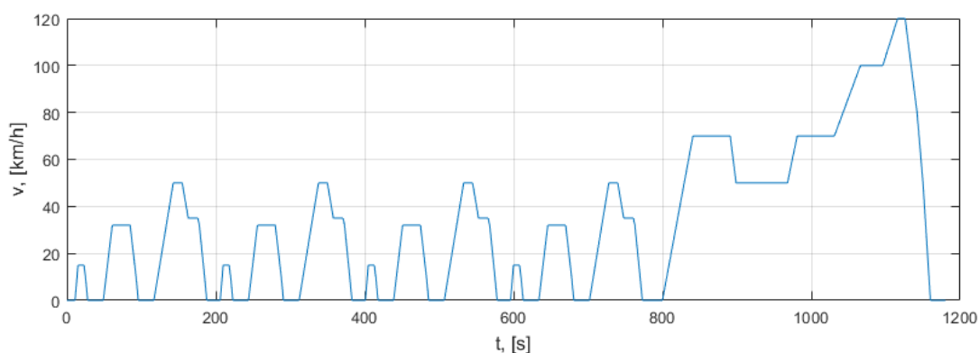
Slika 5.1. Profil brzine NEDC voznog ciklusa
