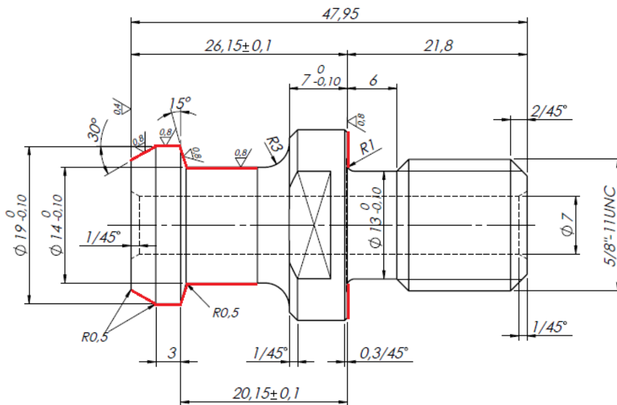
Slika 12. Obradene površine
