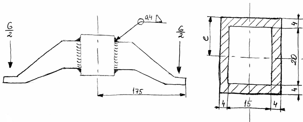
Slika 26. Opterećenje zavara rotacijskog postolja
