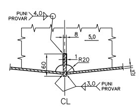
DETALJ "1": M 1:5
