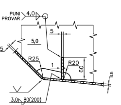
DETALJ "3": M 1:5
