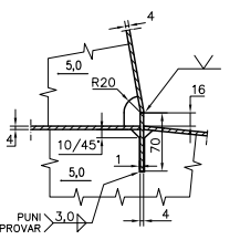
DETALJ "5": M 1:5
