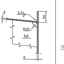
DETALJ "6": M 1:5
