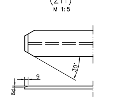
ZAVRŠETAK TRAKE TIP 1 (ZT1) M 1:5
