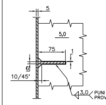
DETALJ "7": M 1:5
