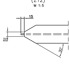
ZAVRŠETAK TRAKE TIP 2 (ZT2) M 1:5
