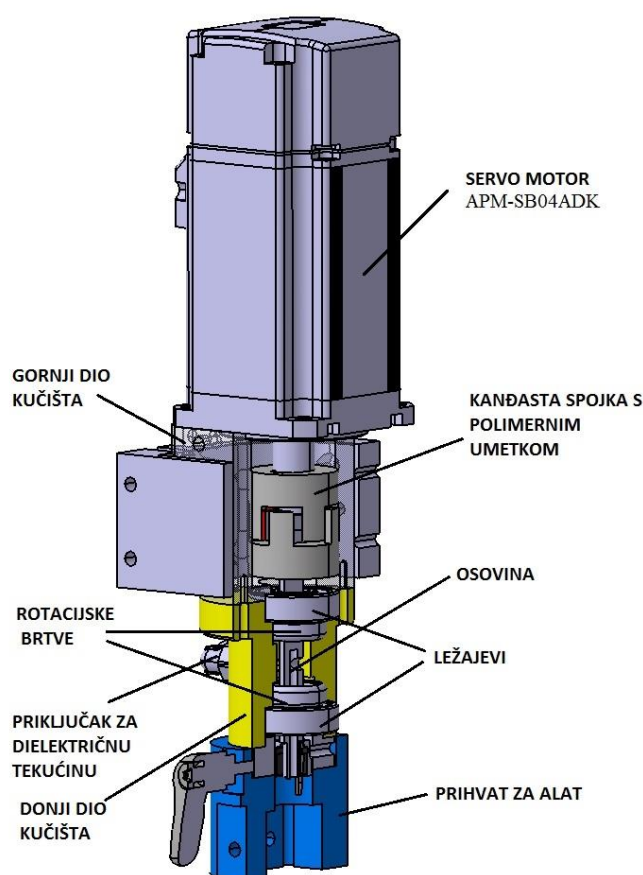
Slika 39. Sklop kućišta
