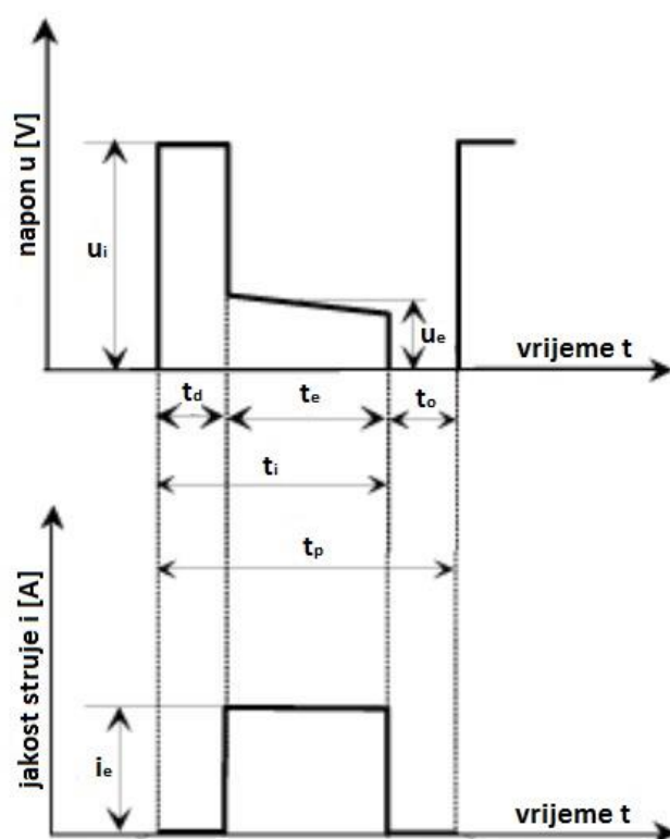
Slika 6. Dijagram napona i jakosti struje za vrijeme električnog pražnjenja [6]
