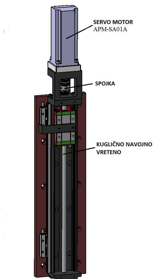
Slika 35. Prigon osi Z
