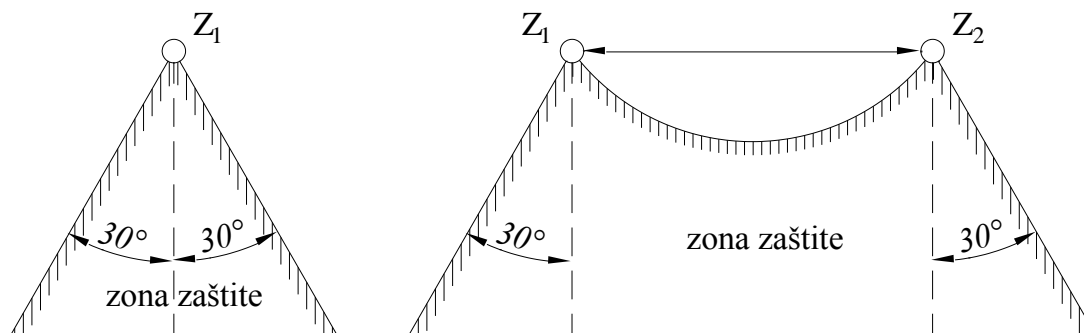
Slika 2.7. Zaštitna zona zaštitne užadi [4]
