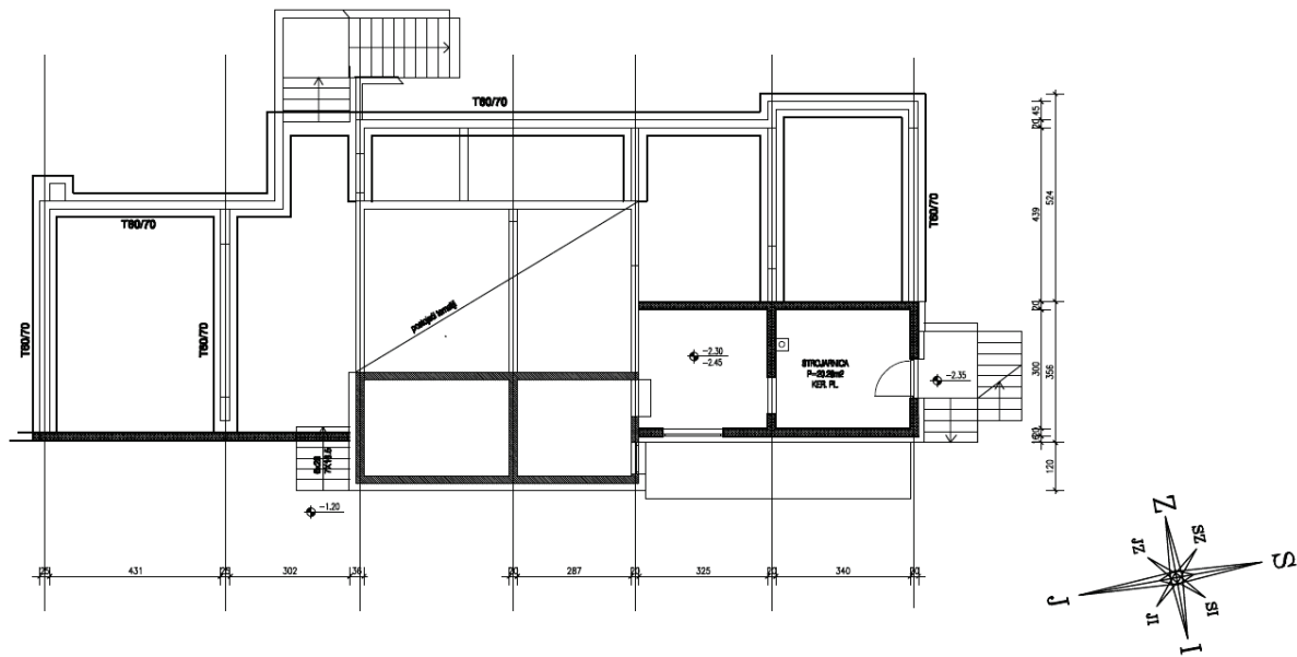
Slika 11: Tloct podruma
