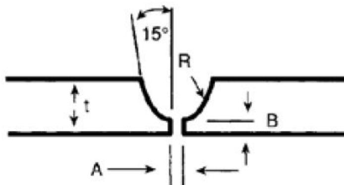
Slika 18. Sučeljeni jednostrani "U" spoj limova [15]
