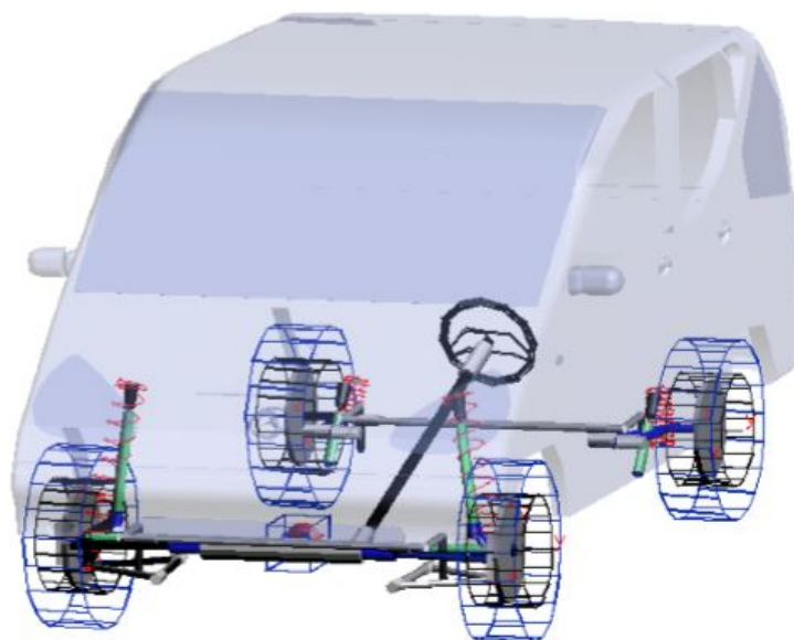
Slika 23. Simulacijski model za Mercedes-Benz A-klasom [11]
