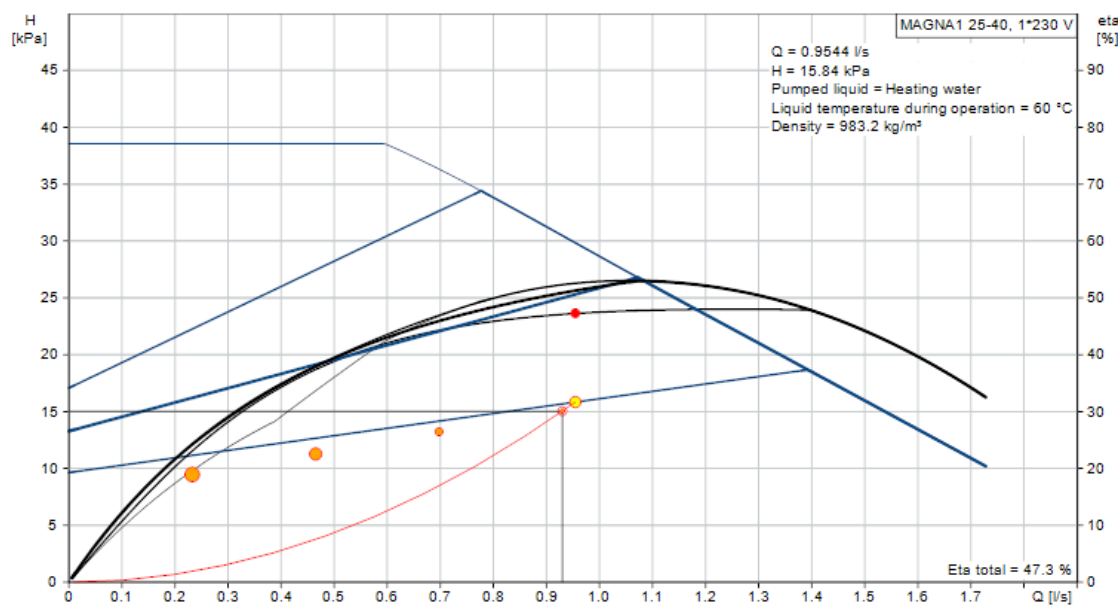
Slika 23. Dijagram radne točke pumpe MAGNA1 24-40
