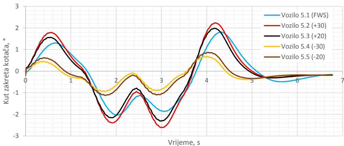
Slika 59. Kut zakreta prednjih kotača
