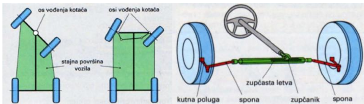
Slika 2. Shema upravljanja zakretnom osovinom (lijevo), zakretanjem rukavca kotača (sredina) i upravljanje zakretanjem rukavca - M1 kategorija (desno) [4]
