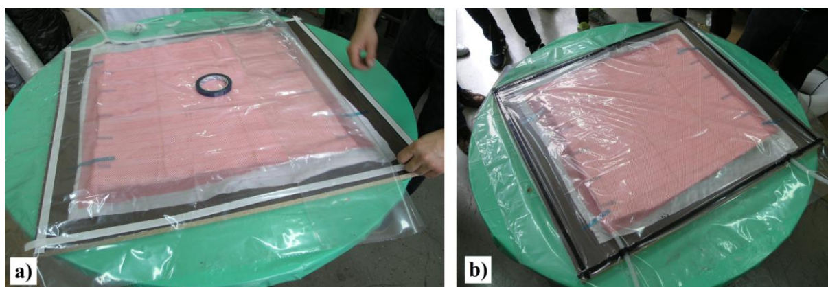
Slika 6.7. Zatvaranje kalupa folijom za brtvljenje
