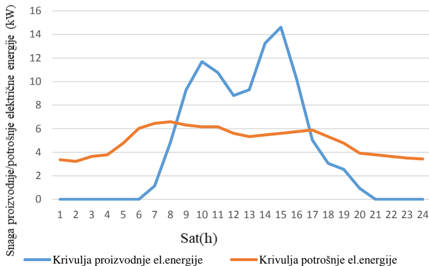
Slika 11. Odnos krivulja potrošnje i proizvodnje el.energije za ljetni dan
