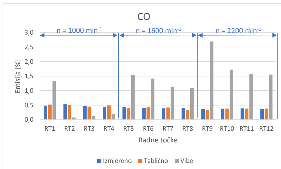
Slika 22. Usporedba emisija CO po radnim točkama
