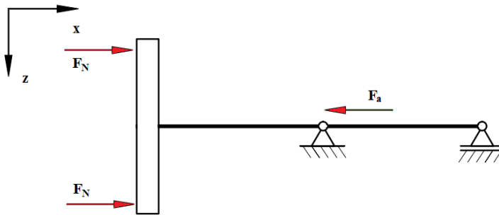
Slika 27. Opterećenja na vratilu V_3 u z - x ravnini
