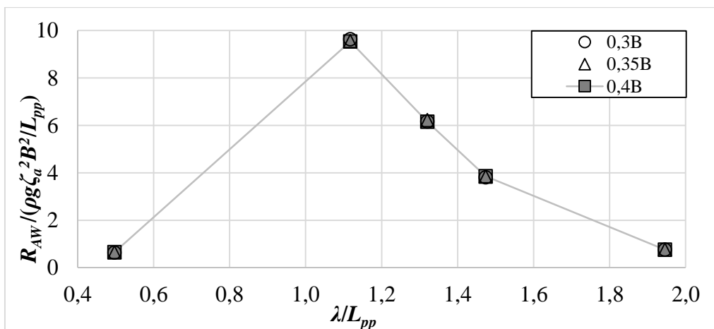
Slika 45. Utjecaj radijusa tromosti mase oko osi x na dodatni otpor na valovima kod \beta=150^\circ za KCS pri Fr = 0,26
