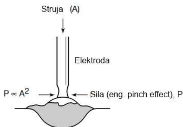
Slika 8. „Pinch efekt“ [15]
