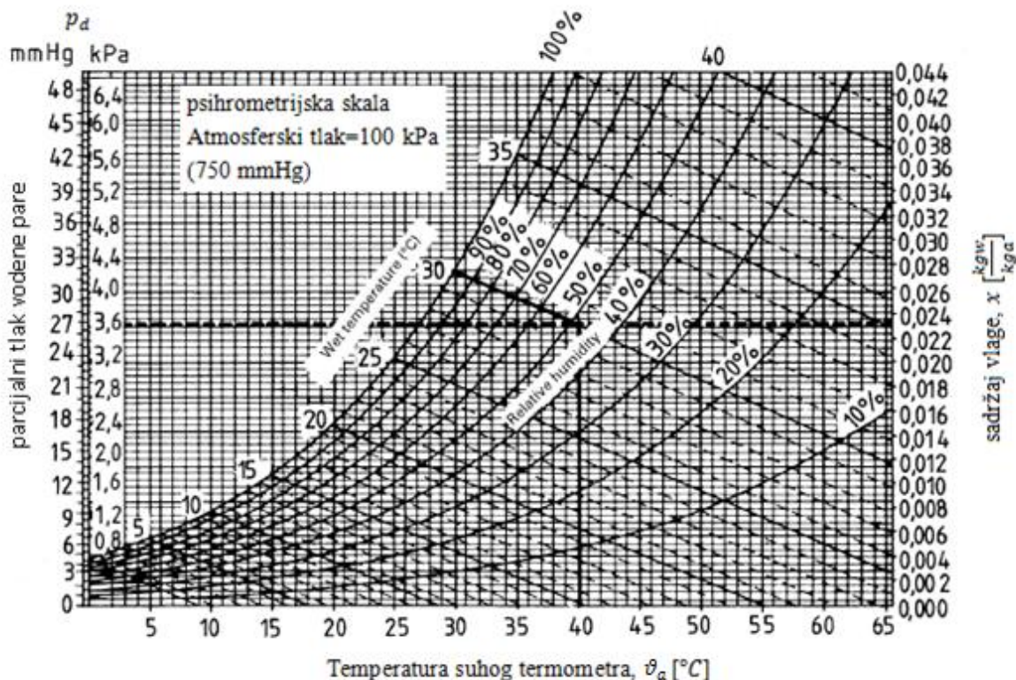
Slika 13 – Psihrometrijski grafikon [11]
