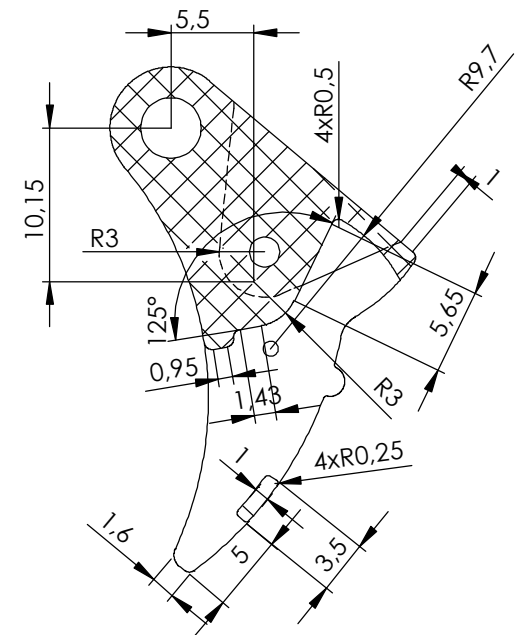
Presjek B-B
