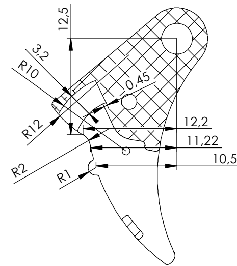
Presjek A-A
